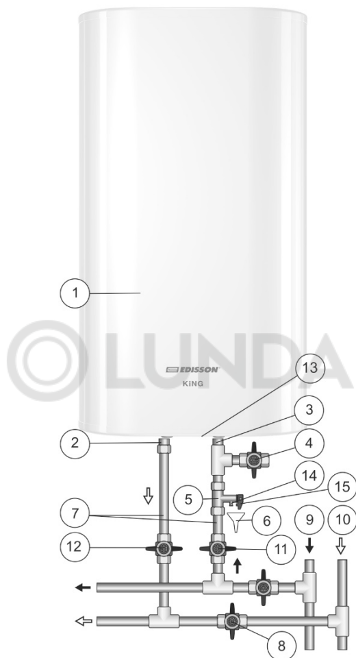
Рисунок 1. Схема подключения ЭВН к водопроводу сверху и снизу
