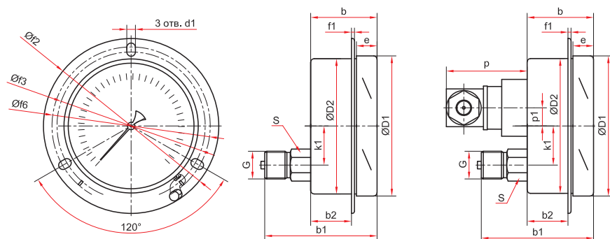
Эксцентрическое присоединение с передним фланцем (ТМж, ТМж с подств.)
