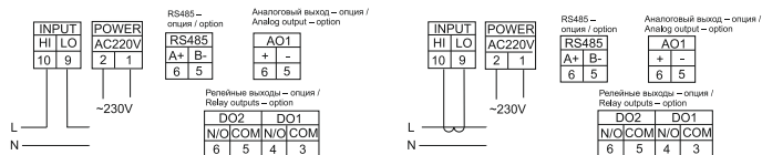
c) схема подключения 1-ф. амперметра при I \leq 5\text{ А} / connection diagram of 1-ph. ammeter at I \leq 5\text{ A}
