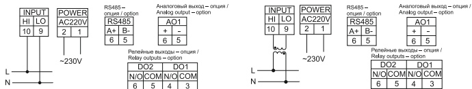
a) схема подключения 1-ф. вольтметра при U \leq 600\text{ В} / connection diagram of 1-ph. voltmeter at U \leq 600\text{ V}
