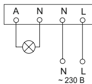
Рисунок 17 – Схема подключения датчика ДД 201
