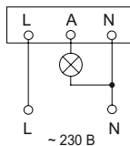
Рисунок 18 – Схема подключения датчика ДД 301
