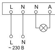
Рисунок 16 – Схема подключения датчика ДД 026, ДД 401
