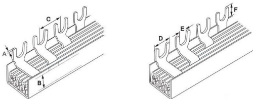
Рисунок 3 – Шина типа FORK 3P 63, 100 А
