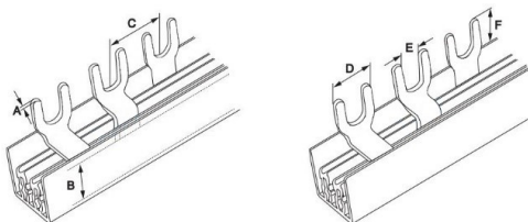
Рисунок 2 – Шина типа FORK 2P 63, 100 А
