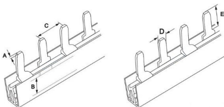
Рисунок 5 – Шина типа PIN 1P 63, 100 А
