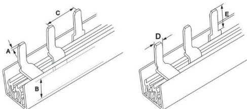
Рисунок 6 – Шина типа PIN 2P 63, 100 А
