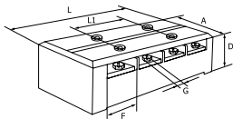
Рис. 2 - Клеммный терминал серии ТС
