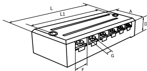
Рис. 1 - Клеммный терминал серии ТВ
