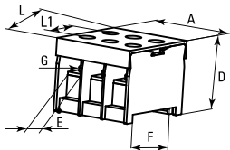
Рис. 3 - Клеммный терминал серии БЗД
