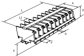
Рис. 4 - Клеммный терминал серии ТК
