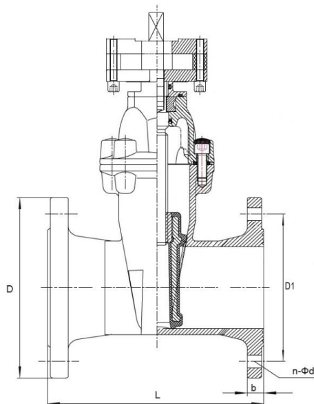
Рисунок 2 - Размеры
