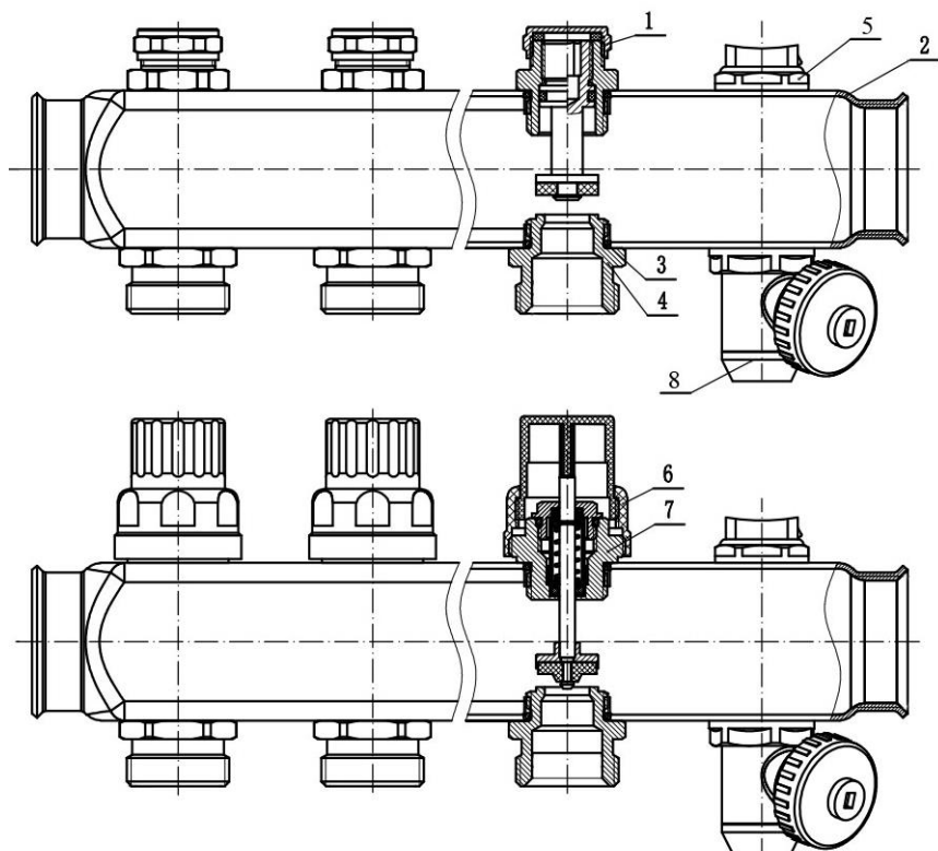
Рисунок 2 – Деталировка
