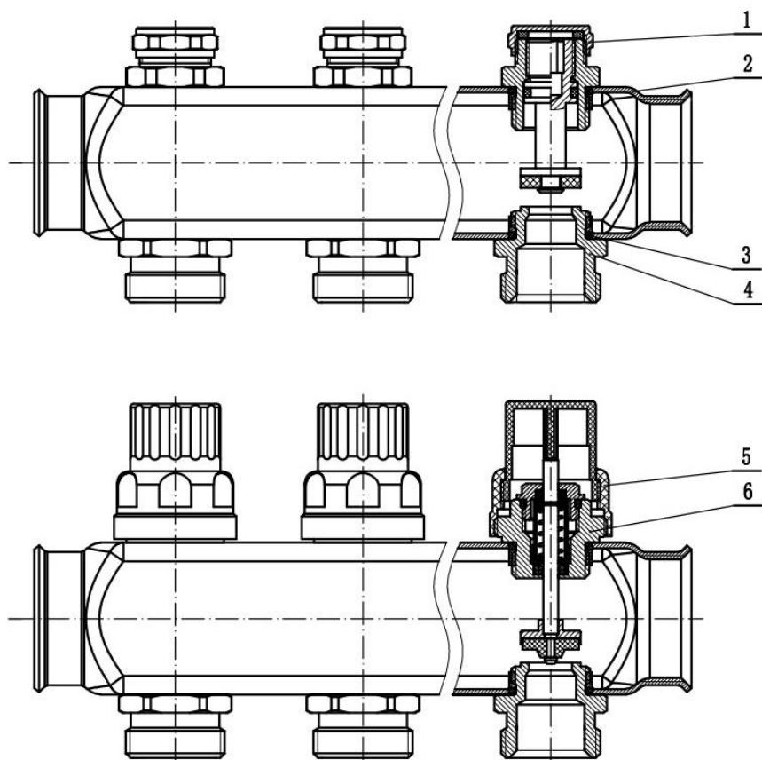
Рисунок 2 – Деталировка
