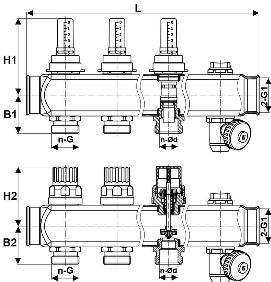
Рисунок 3 – Размеры
