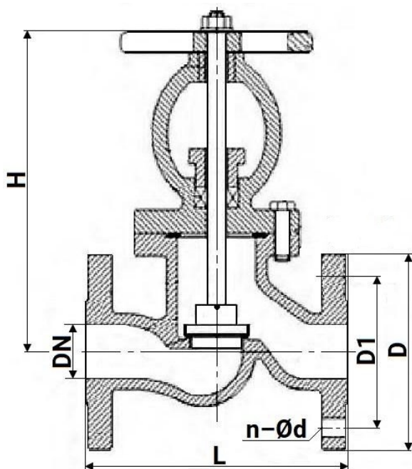
Рисунок 2 – Размеры
