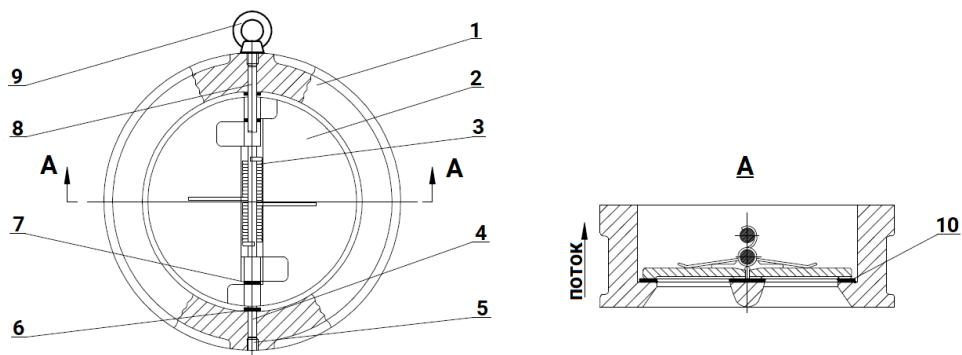
Рисунок 2 – Деталировка
