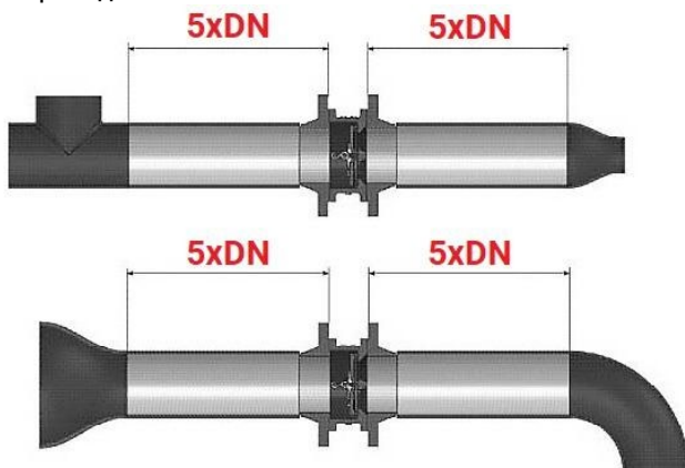
Рисунок 4 – Схемы установки
