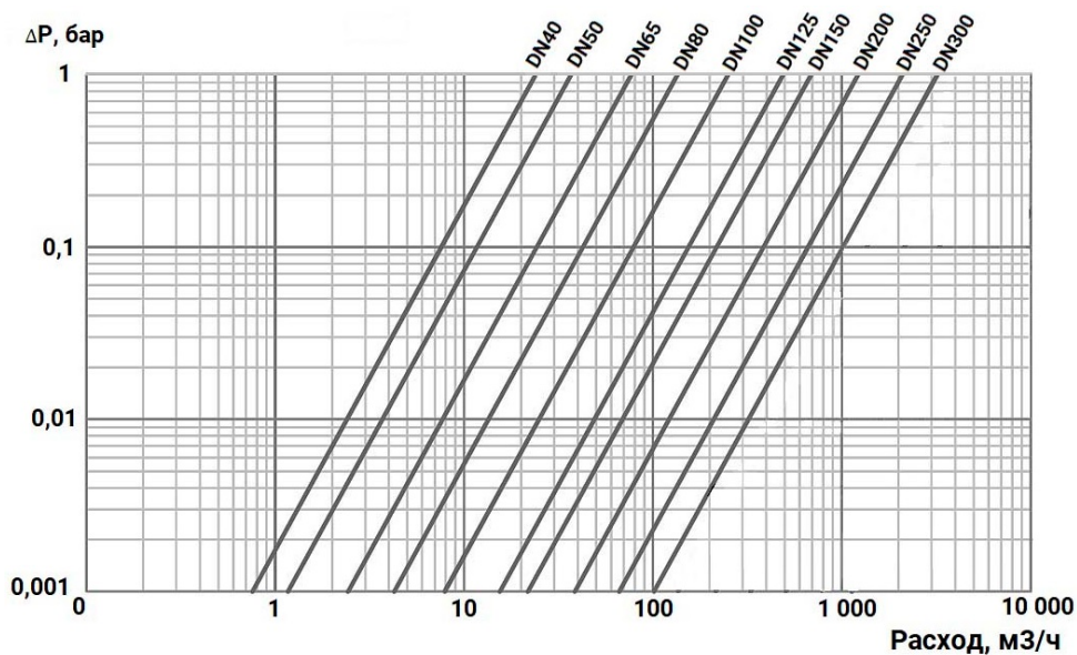
Рисунок 1 – Диаграмма потери давления
