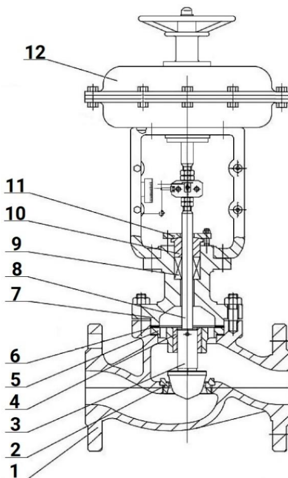
Рисунок 2 – Деталировка
