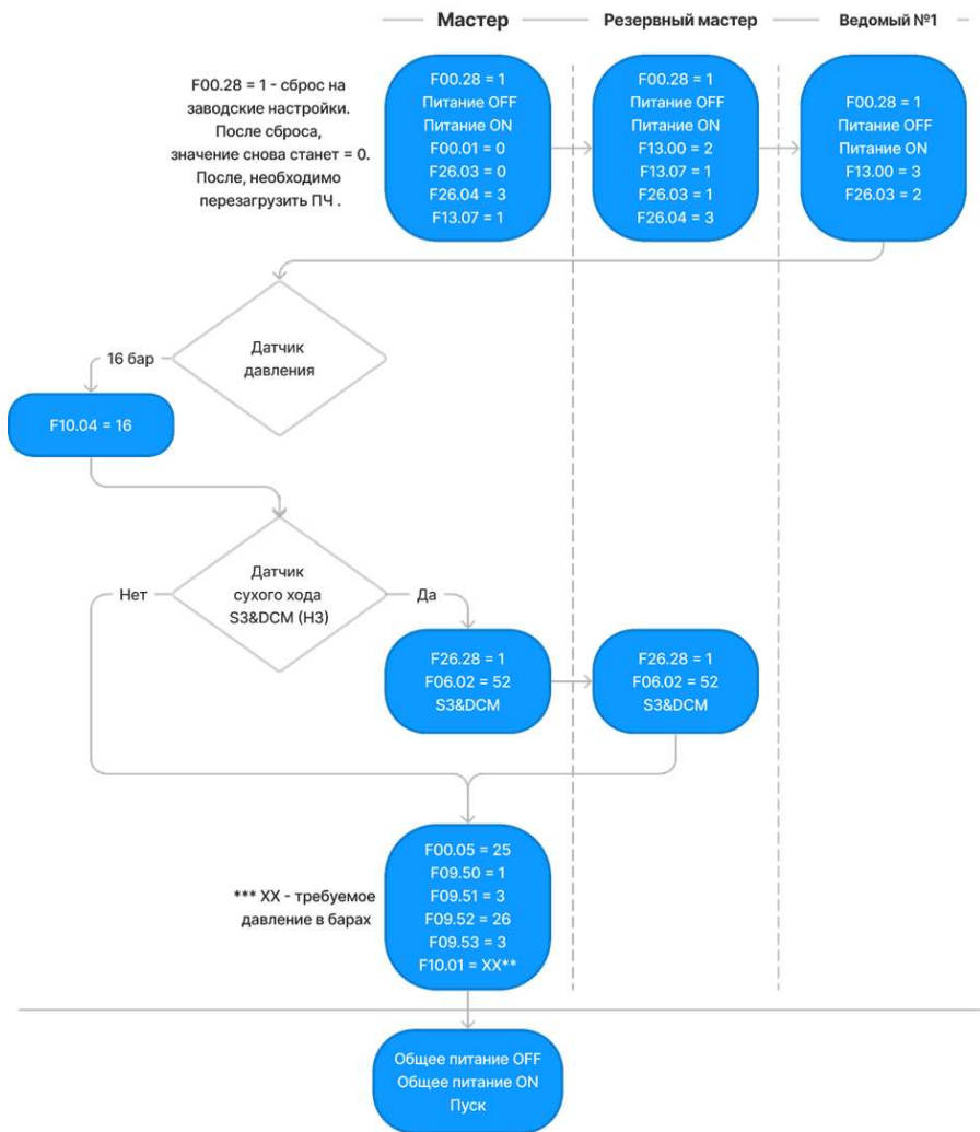
Рис. 13 Пример настройки 3-х насосной станции
