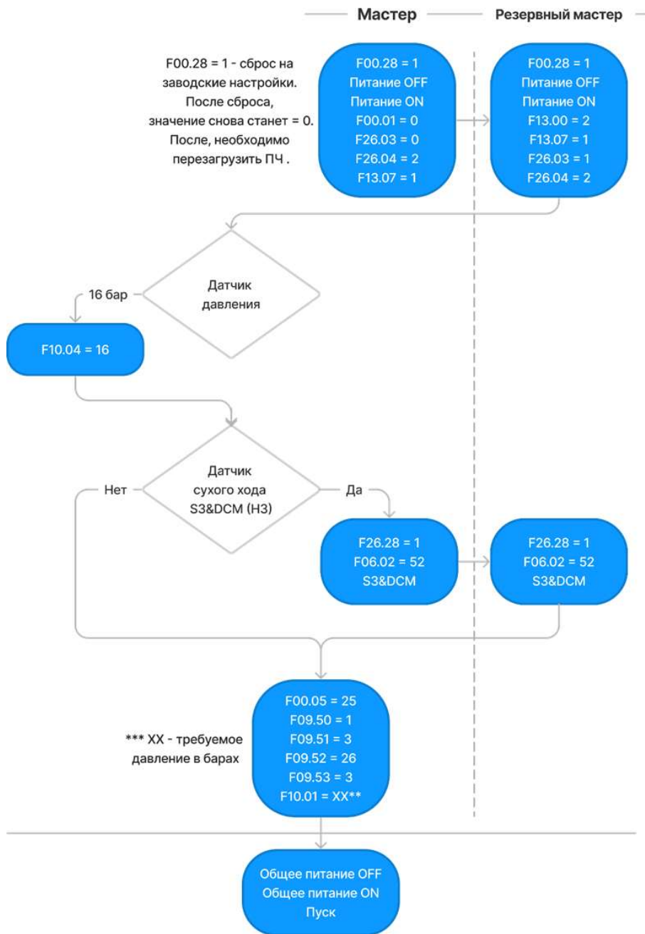
Рис. 12 Пример настройки 2-х насосной станции
