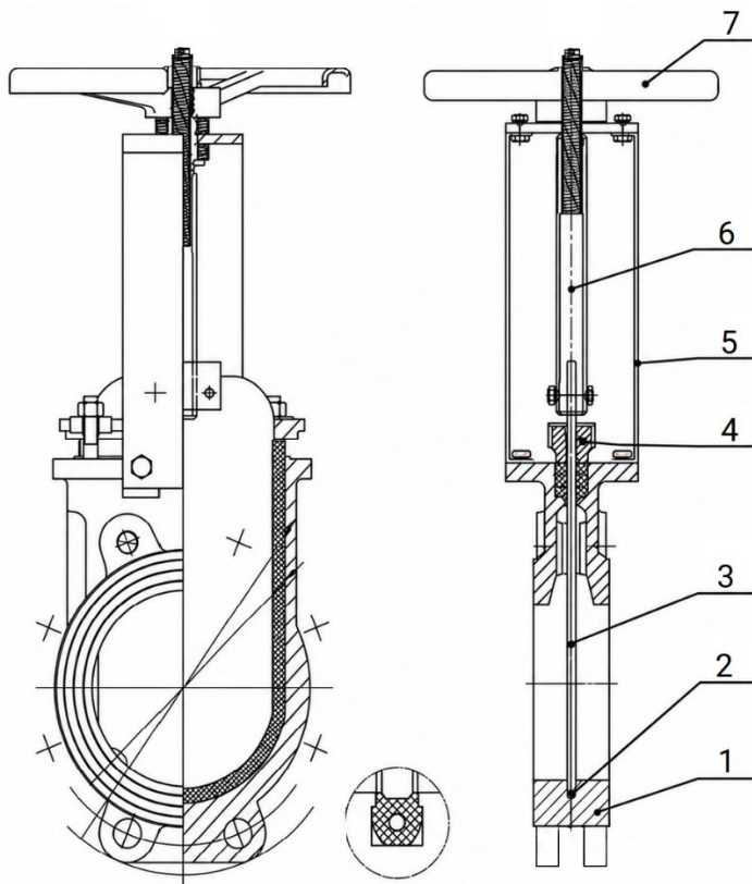
Рисунок 2 – Составные части изделия
