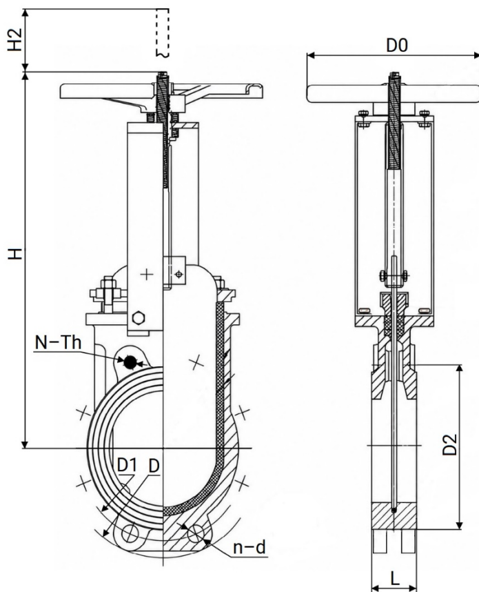
Рисунок 3 – Размеры изделия
