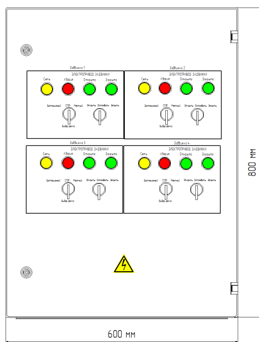
Рис. 1. Габаритные размеры ШАУ-3
