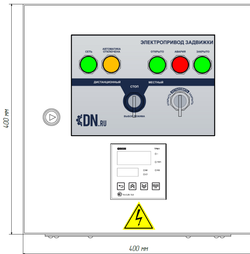
Рис. 1. Габаритные размеры ШАУ-3
