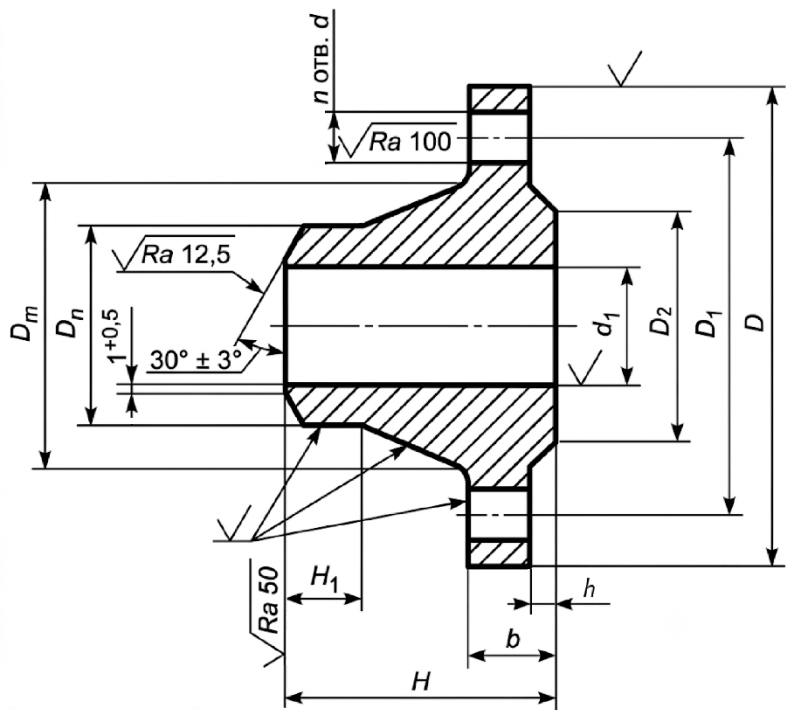
Рисунок 2 – Размеры изделия
