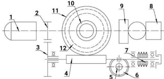
Рисунок 4 – Элементы электропривода
