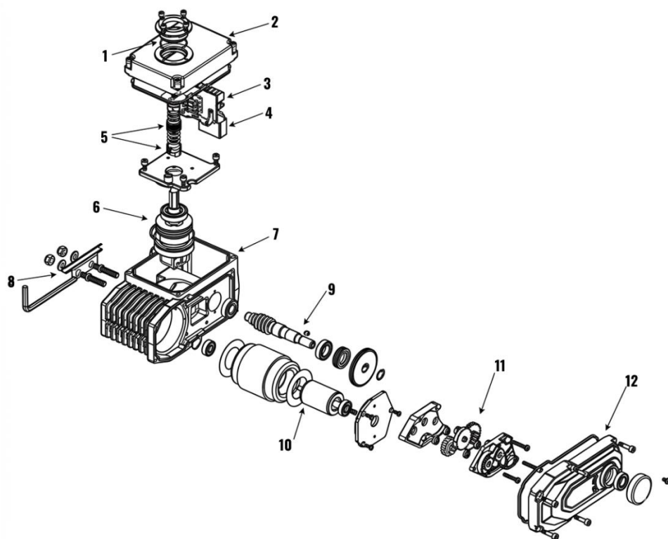
Рисунок 2 – Основные детали
