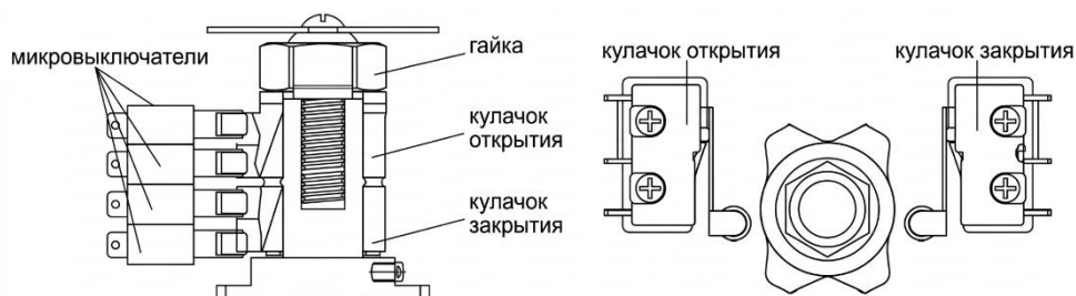
Рисунок 7 – Концевые выключатели
