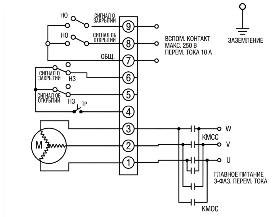
Рисунок 5 — Схема подключения электропривода на 380 В
