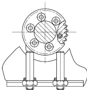
Рисунок 8 – Механический ограничитель
