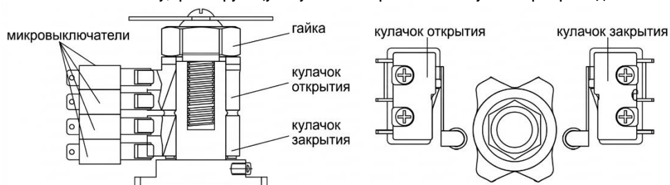
Рисунок 6 – Концевые выключатели
