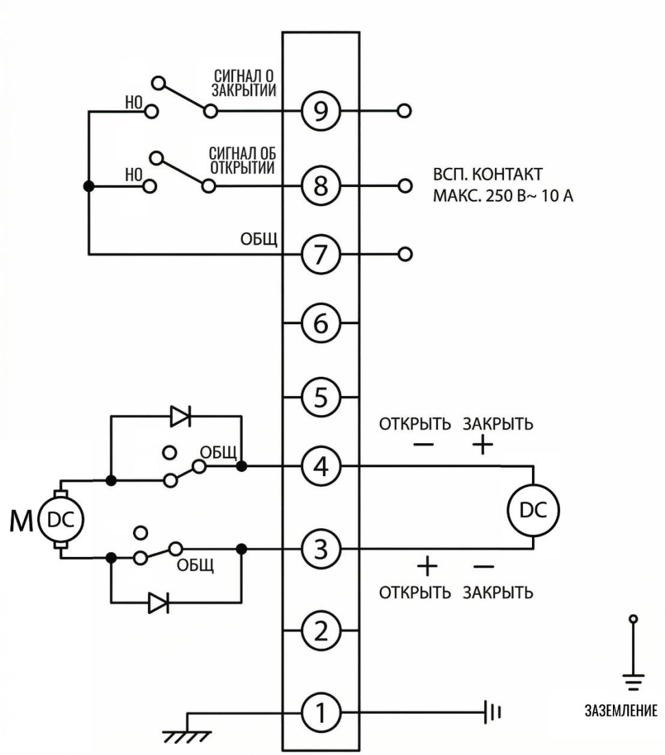
Рисунок 5 – Схема подключения электропривода на 24 В
