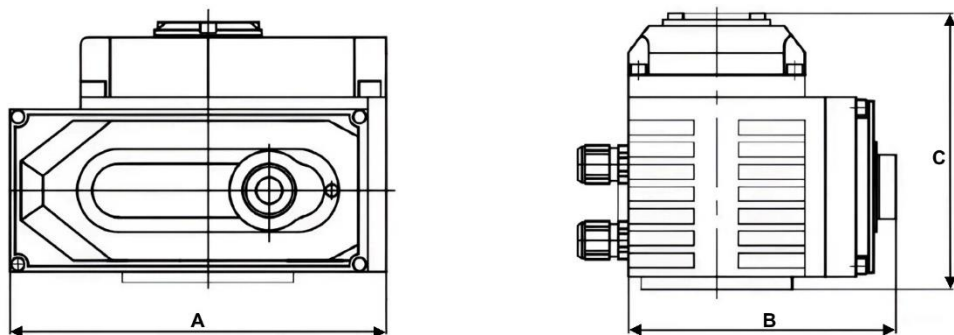
Рисунок 3 – Размеры электропривода 30Нм
