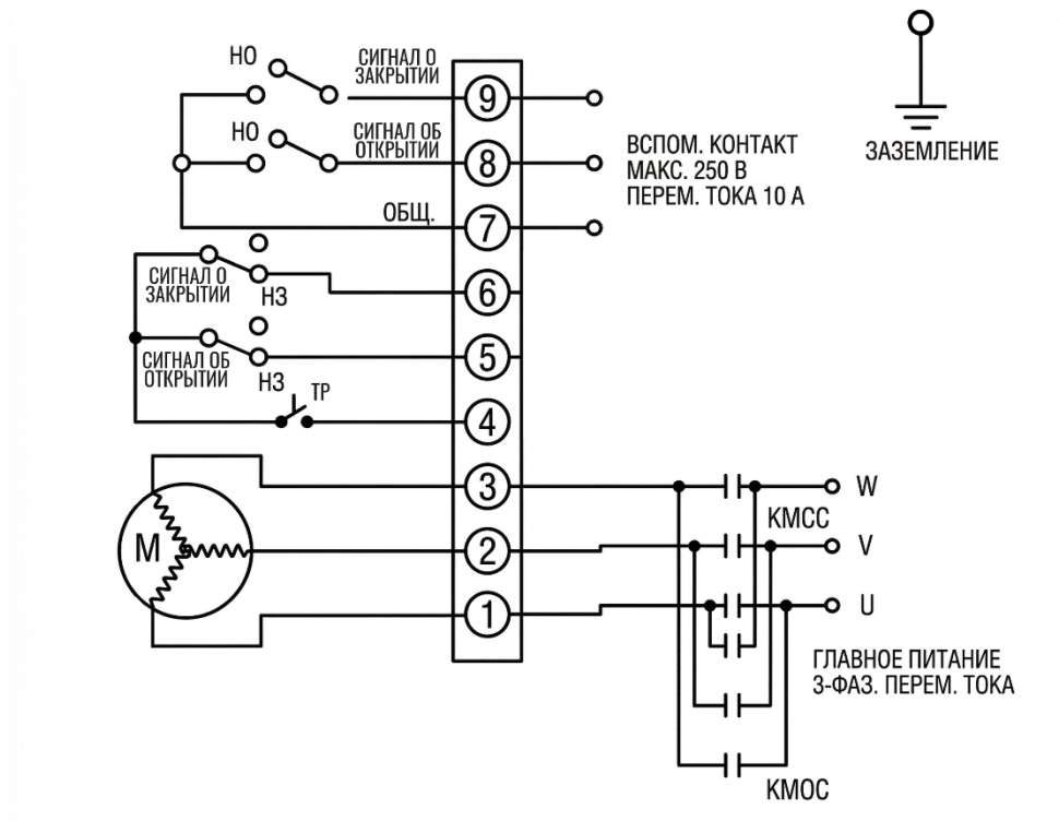
Рисунок 4 — Схема подключения электропривода на 380 В
