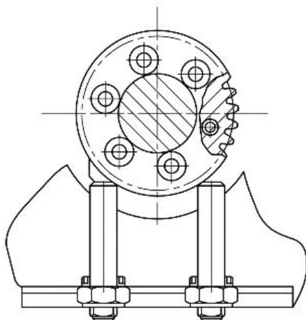
Рисунок 7 – Механический ограничитель
