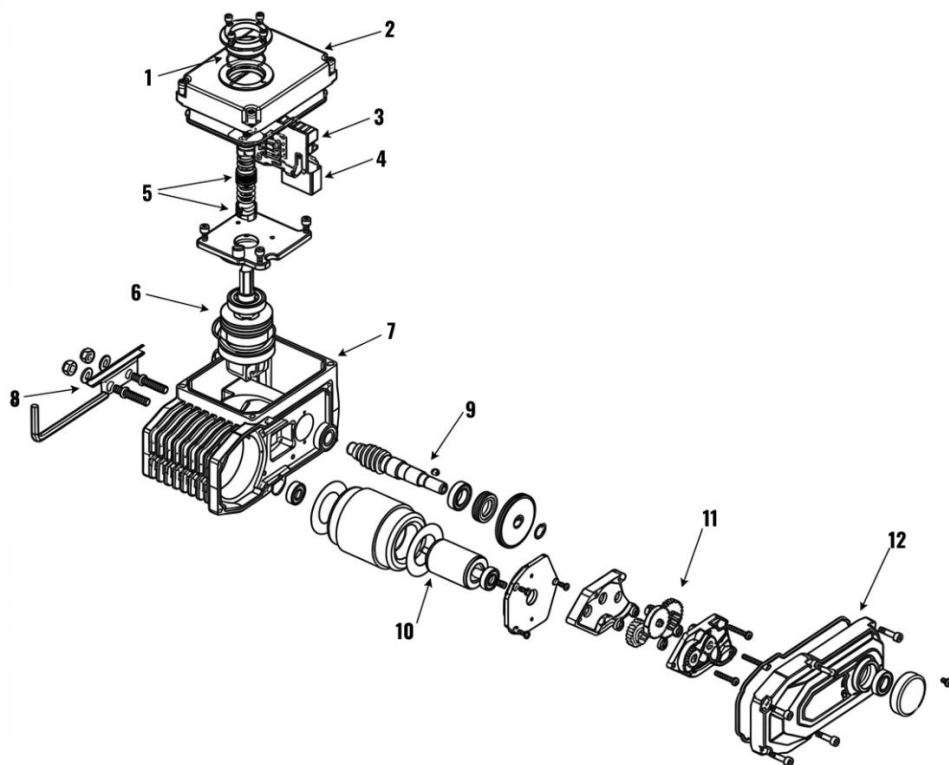
Рисунок 2 – Основные детали
