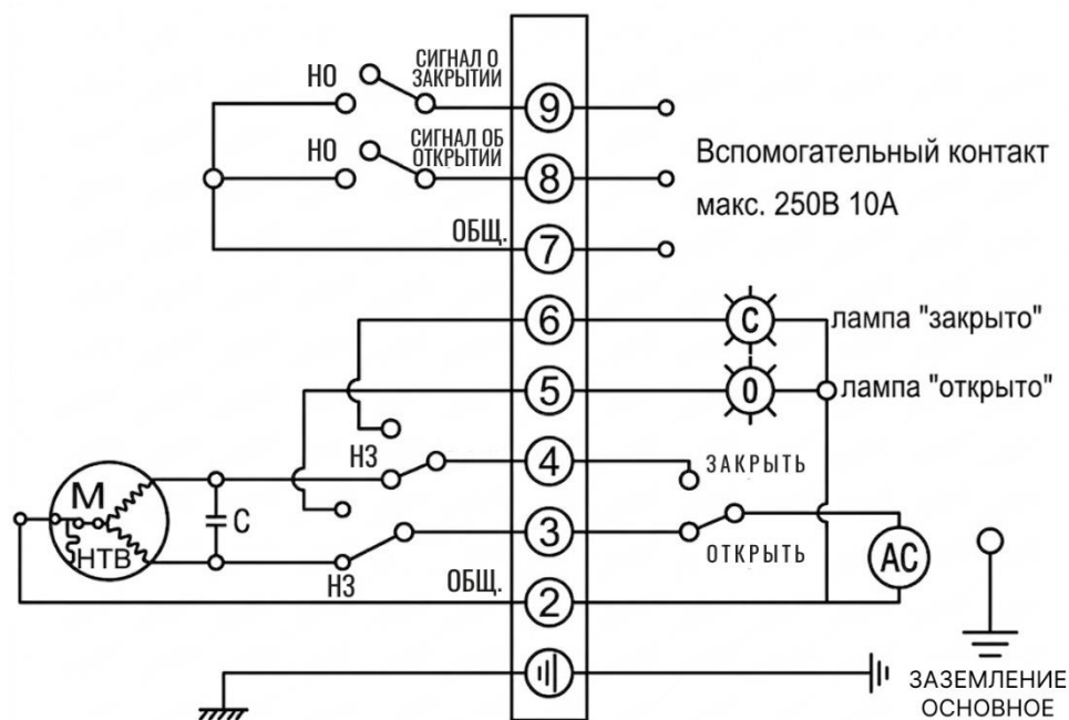
Рисунок 3 – Схема подключения электропривода на 220 В
