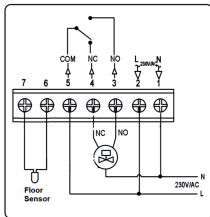
Подключение электропривода
