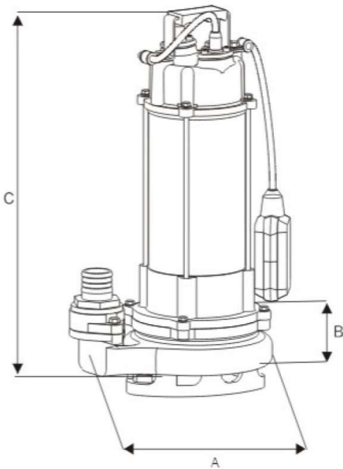
Габаритные размеры
