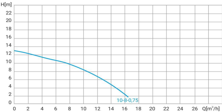
Диаграмма характеристик
