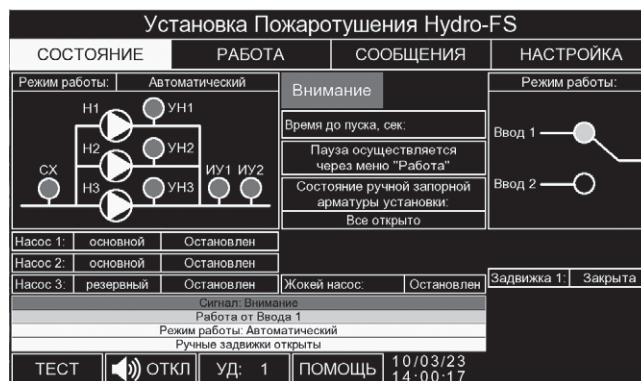
Рис. 14 Меню «Состояние»
