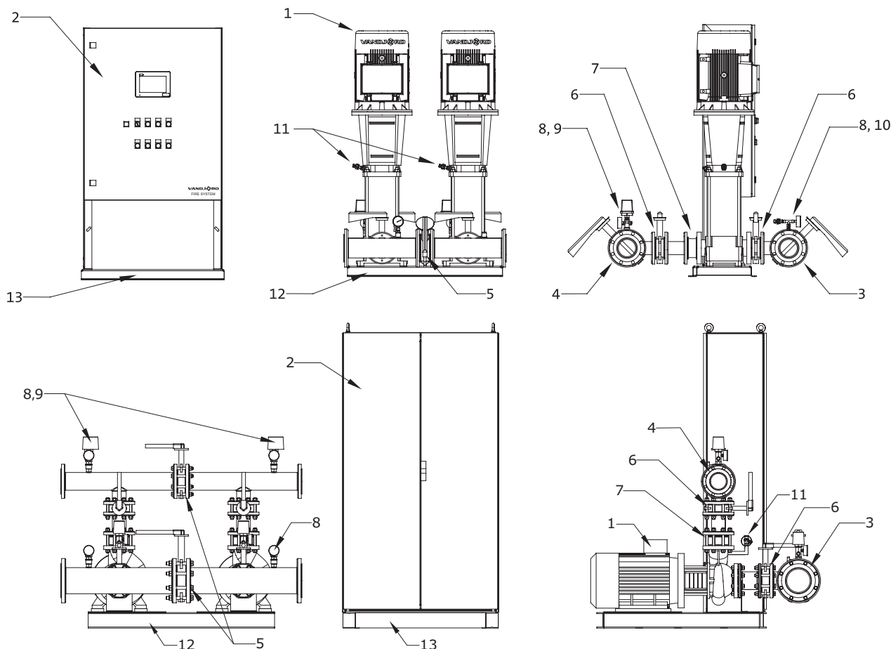
Рис. 4 Внешний вид установки Hydro-FS-A на примере системы с одним основным и одним резервным насосами CRV или NB(G)V
