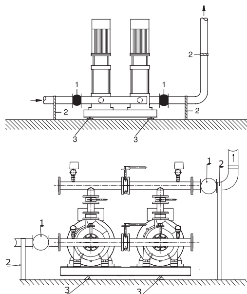
Рис. 6 1 – Компенсаторы (упругие соединительные патрубки) для труб; 2 – Жесткие опоры для крепления труб; 3 – Виброизолирующие опоры
