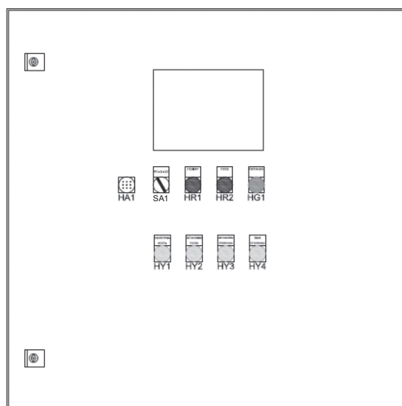
Рис. 11 Прибор управления пожарной Control MX
