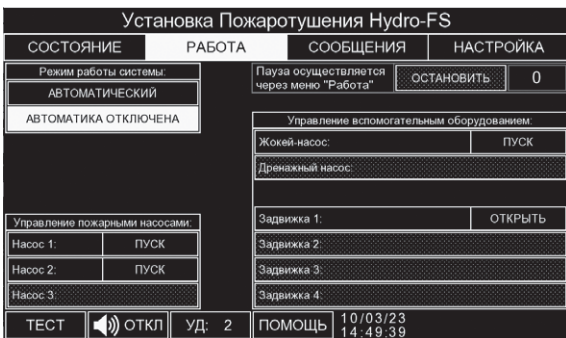
Рис. 16 Меню «Работа»
