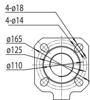
Фланец напорного патрубка насоса DN50 PN6/PN10
