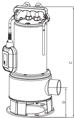
APV.40/45/50B (без охлаждающего кожуха)
