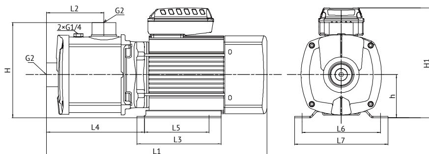
Рисунок 8 – Размеры насосов CM 25
