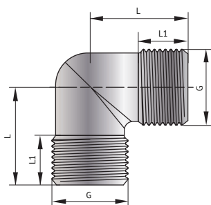
Угол Н
