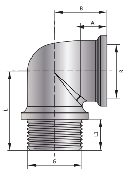
Угол НВ с упором
