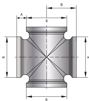
Крестовина В
