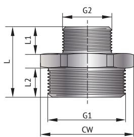
Ниппель редукционный
