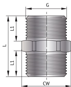
Ниппель
