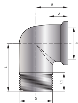
Угол НВ
