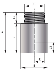
Удлинитель НВ
