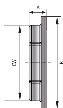
Контргайка с бортиком
