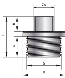
Заглушка Н с квадратом
