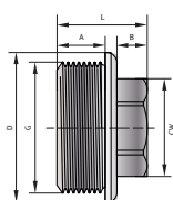
Заглушка Н
