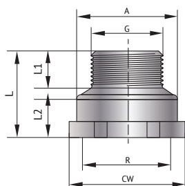
Переходник НВ
