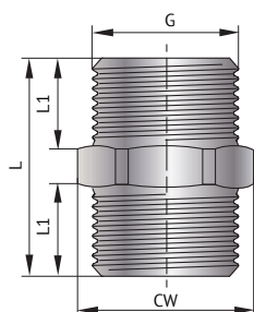
Ниппель удлинённый
