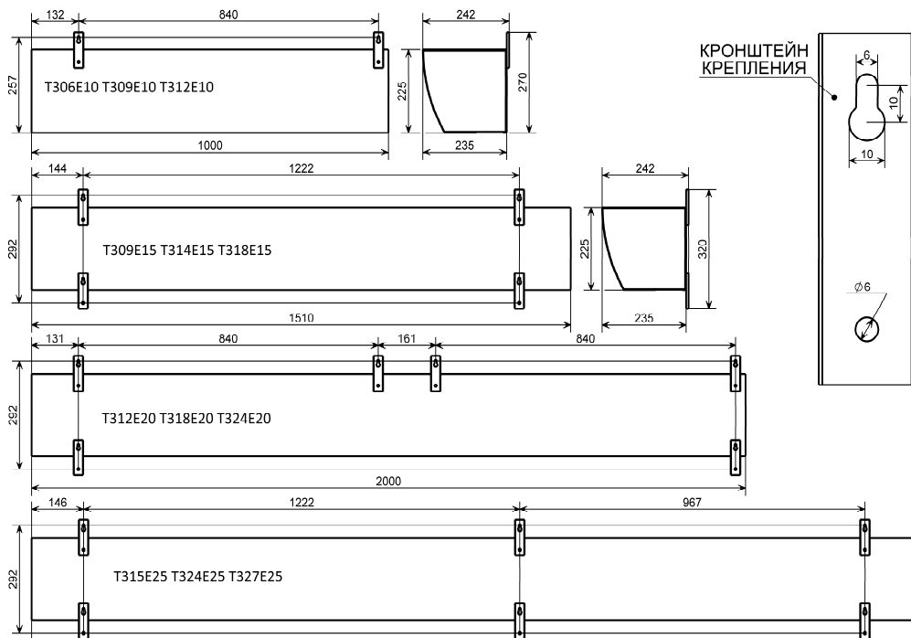
Рис. 2. Габаритные и установочные размеры приборов
