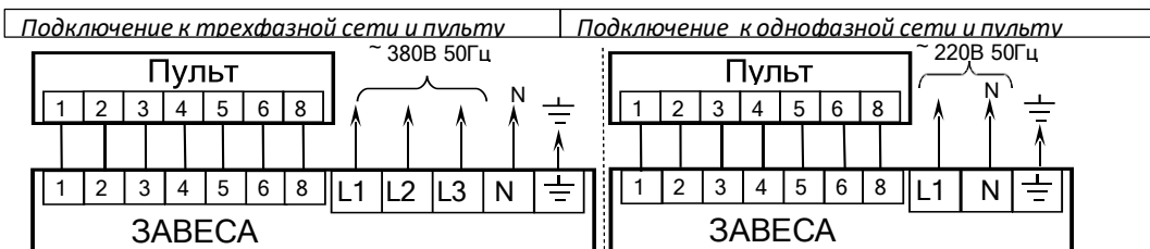
Рис. 3. Схемы подключения завес к электросети и пульту управления
