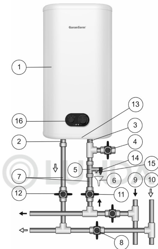
Рисунок 1. Схема подключения ЭВН к водопроводу сверху и снизу
