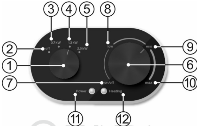
Рисунок 2. Механическая панель управления
