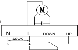
3-позиционный тип
