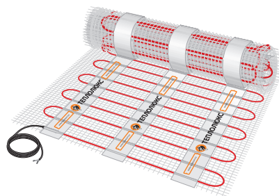
Двужильный мат «ТЕПЛОЛЮКС» TROPIC MHN
