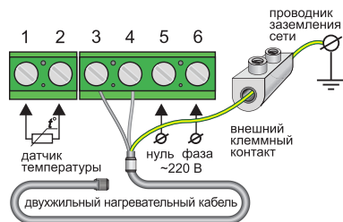
Схема подключения к 3-х проводной электрической сети
