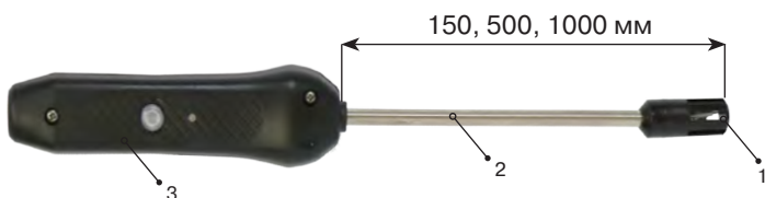
Рис.А.8 Смарт-зонд влажности и температуры (СЗВЛ, СЗВЛП)
