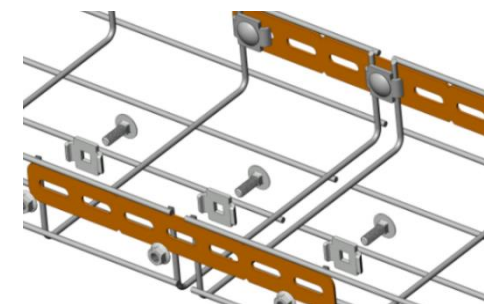
Сборка конструкций кабеленесущих систем
