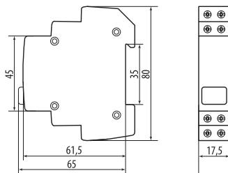
Рисунок 2. Габаритные размеры, мм
