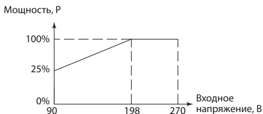
Рисунок 1. График зависимости выходной мощности стабилизаторов от входного напряжения
