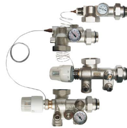
Смесительные узлы
