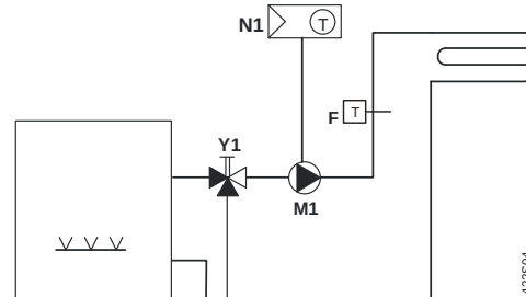
Управление тёплым полом
