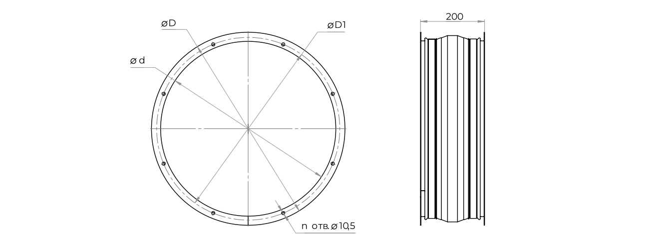
Гибкая вставка «В» типа «фланец-фланец»
