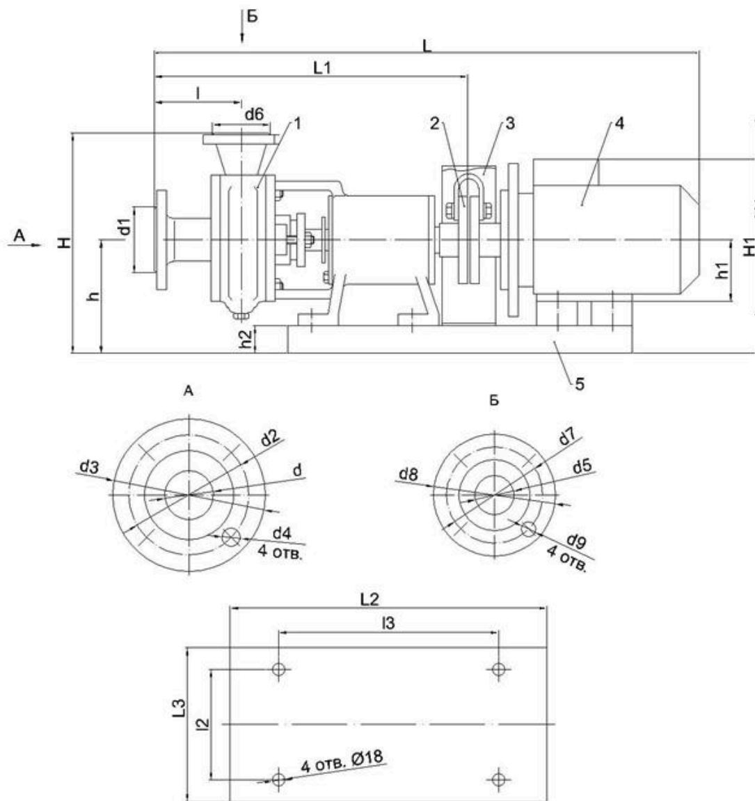
Габаритные и присоединительные размеры насоса 1 - насос; 2 - муфта; 3 - кожух; 4 - электродвигатель; 5 - плита
