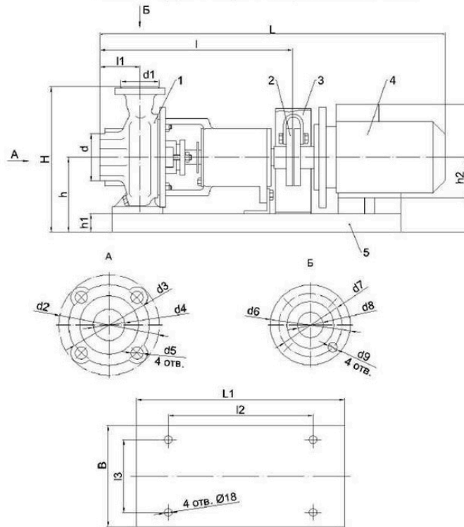
Габаритные и присоединительные размеры 1 - насос; 2 - муфта; 3 - кожух; 4 - электродвигатель; 5 - плата
