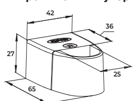
рис. 6 Кронштейн настенный
