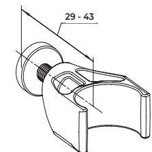
рис. 7 Регулируемый упор
