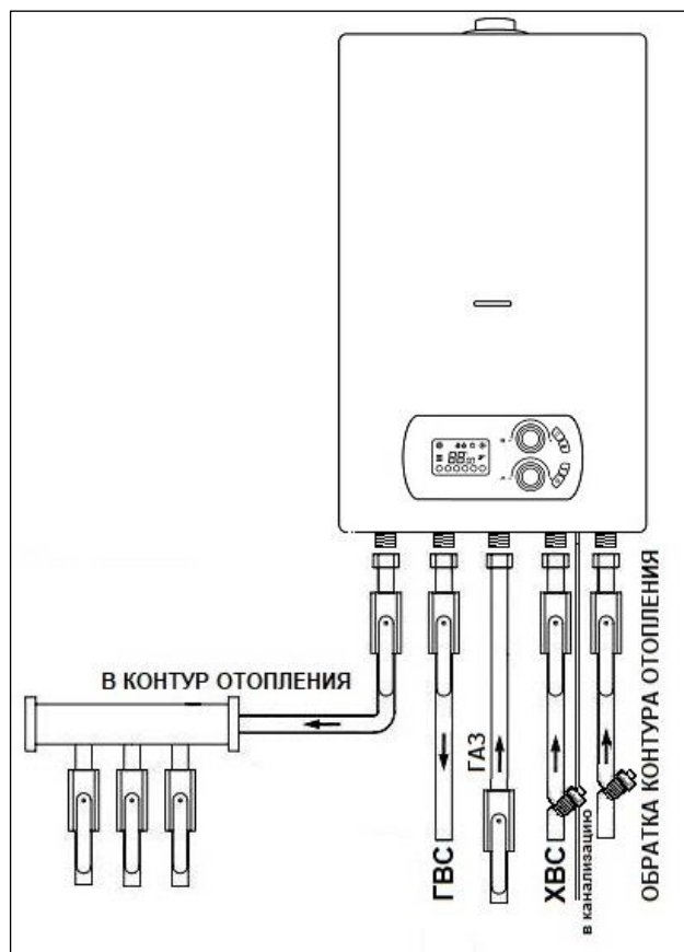
Рис. 6. Схема подключения газового котла
