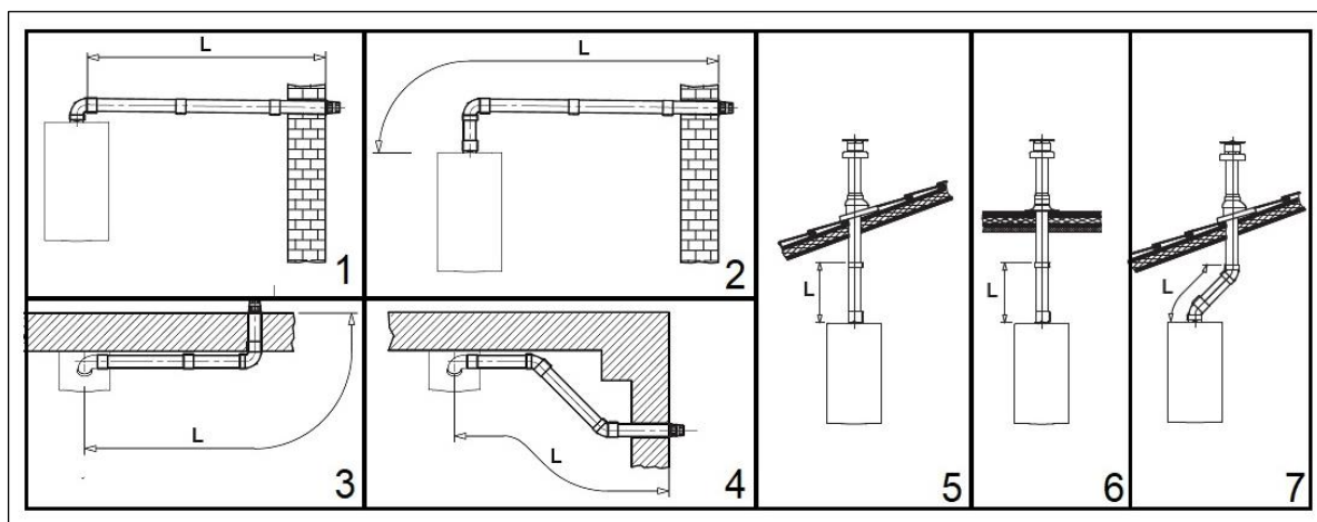
Рис. 5. Монтаж коаксиальной трубы
