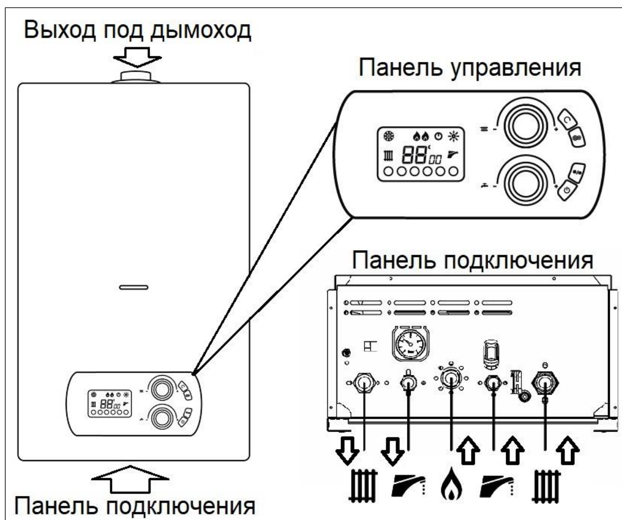
Рис. 1. Общий вид газового котла
