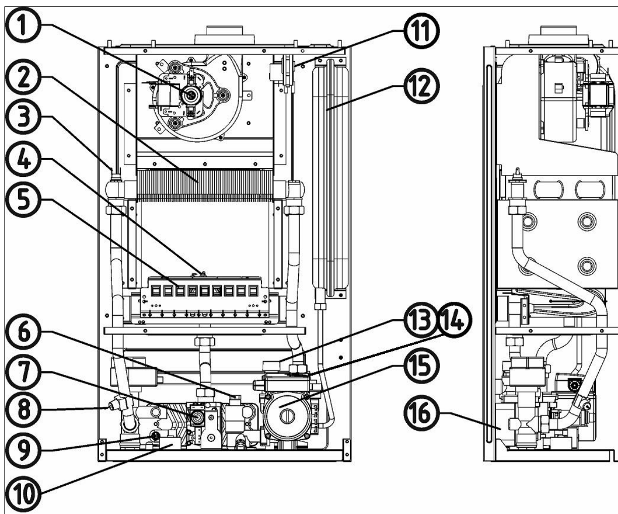
Рис. 2. Внутреннее устройство котла
