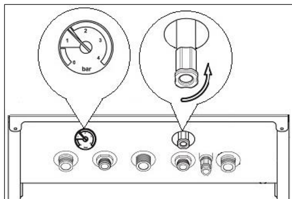
Рис.7 Кран подпитки и манометр
