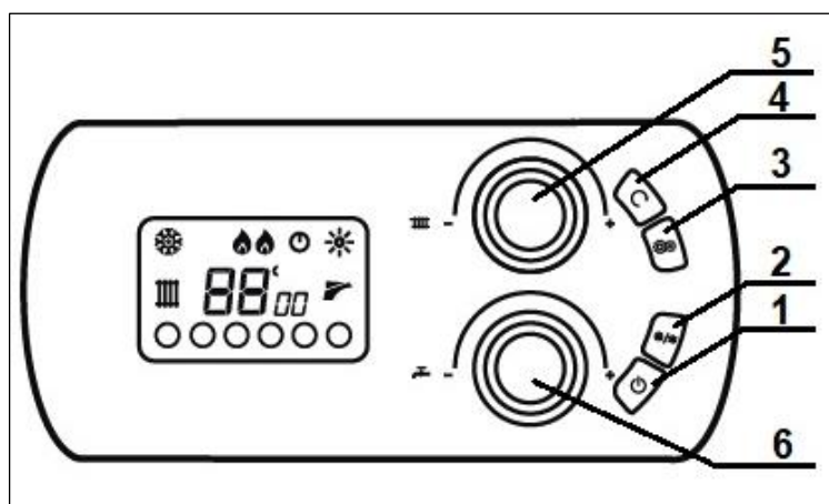
Рис. 8 Панель управления
