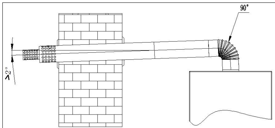
Рис. 4. Монтаж коаксиальной трубы
