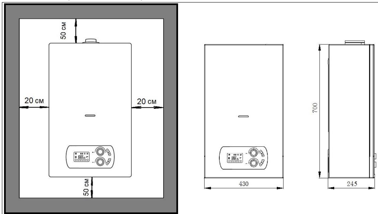
Рис. 3. Минимально допустимые расстояния и габариты котла
