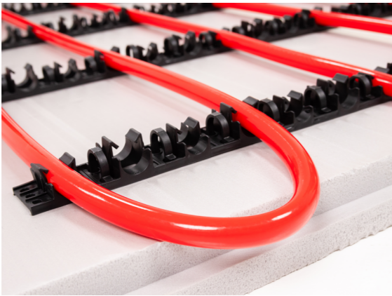
Крепление труб на фиксирующей шине PEXAY
