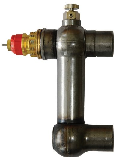
Клапан для двухтрубной системы отопления типа КТК-У2
