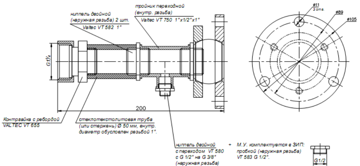
Рис.5б. Монтажный узел юстировочный СЕ-07-05.
