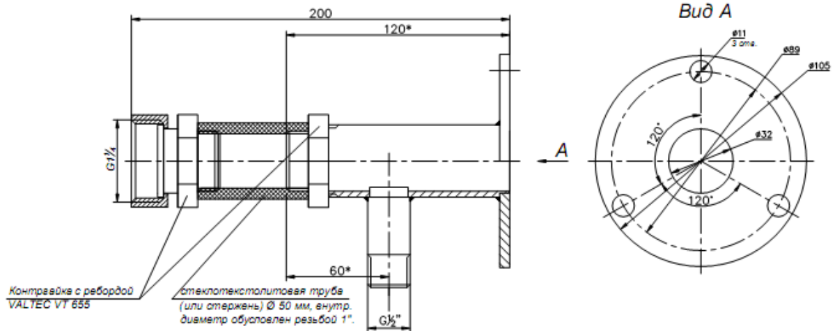
Рис.5а. Монтажный узел СЕ-07-06.
