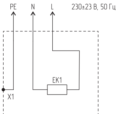
Рисунок 3. Блок-схема электрических узлов и соединений обогревателя в исполнении 60-0010, 60-0011. X1 — контакт подключения защитного заземления. ЕК1 — инфракрасный нагреватель.
