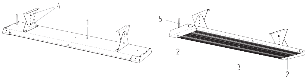
Рисунок 4. Внешний вид и элементы конструкции инфракрасного обогревателя. 1. Кожух. 2. Крышка боковая. 3. Нагревательный элемент. 4. Кронштейн потолочный. 5. Вывод для подключения к электропроводке.
