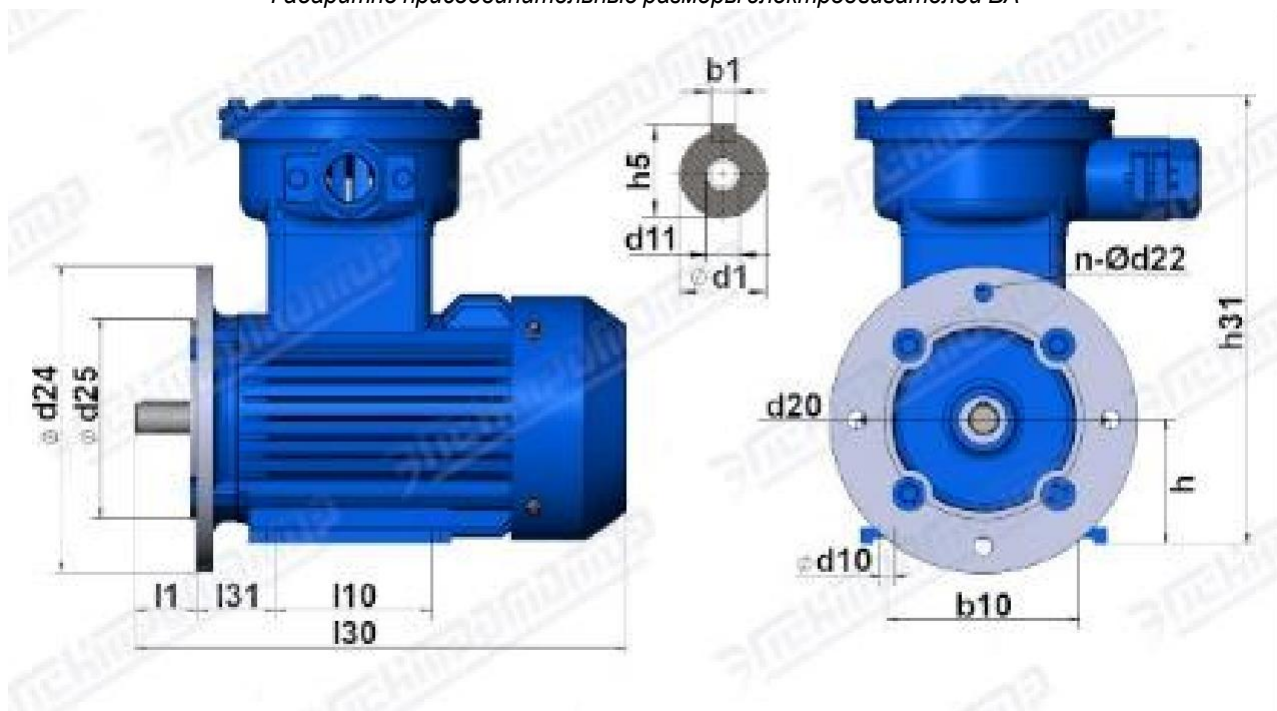
Габаритно присоединительные размеры электродвигателей ВА
