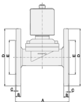
Рисунок 1. Эскиз
