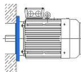
ИСПОЛНЕНИЕ IM 3081
