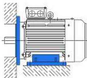
ИСПОЛНЕНИЕ IM 2081
