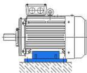
ИСПОЛНЕНИЕ IM 1081
